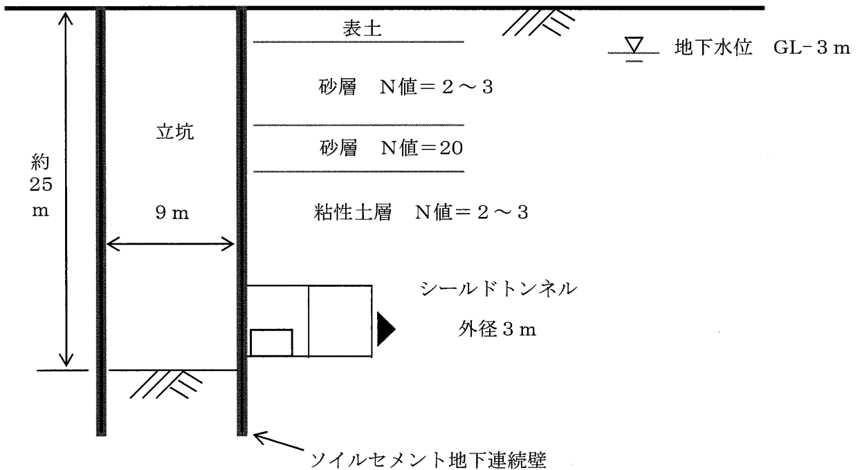
図2 横断面図
