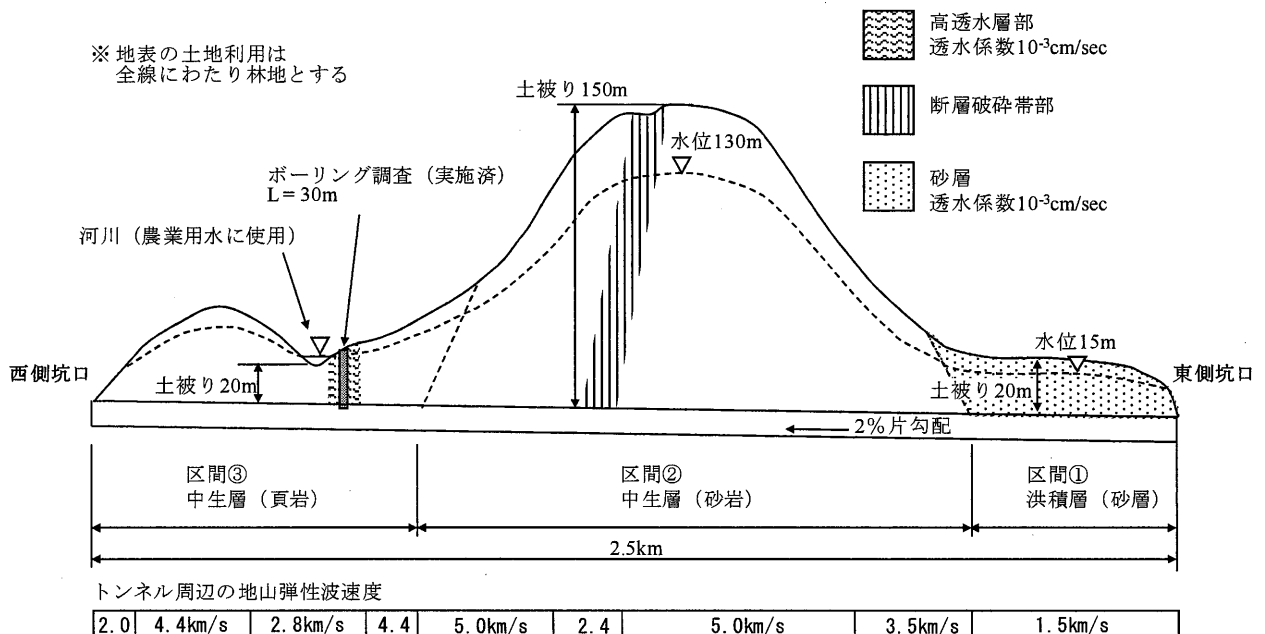
図1 縦断図
